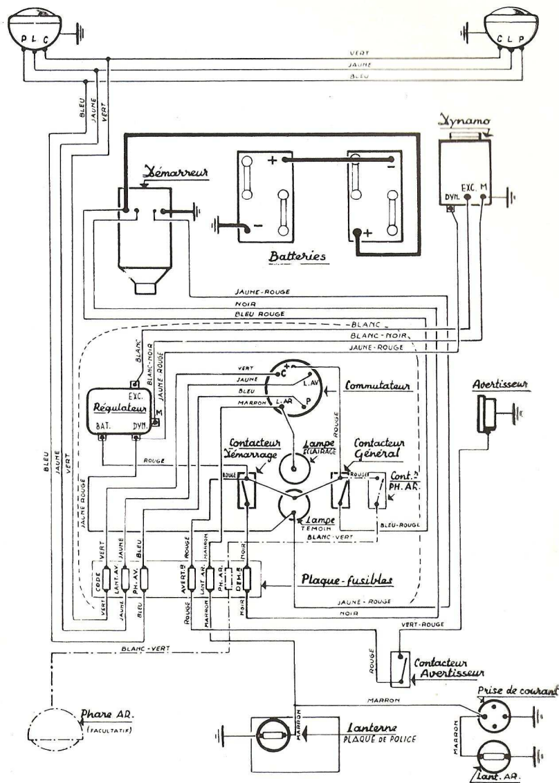
Fig. 42. — Circuit électrique.
